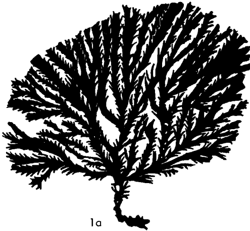
1a Acanthograptus
